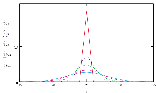
Рис. 3. Изображение графика решения
