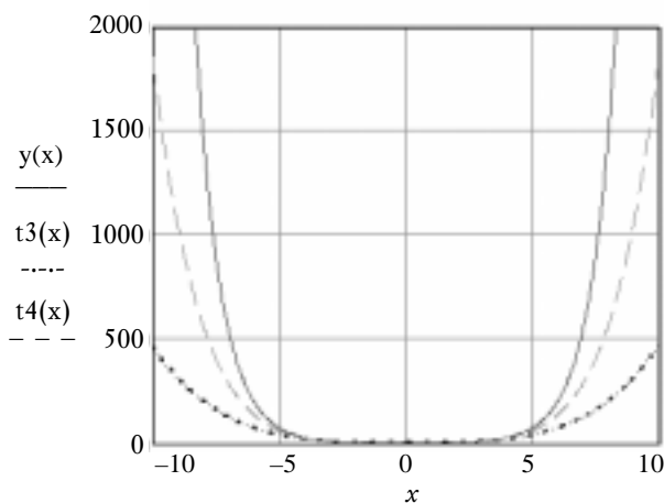
Рис. 2. Аппроксимация функции частичными суммами ряда
