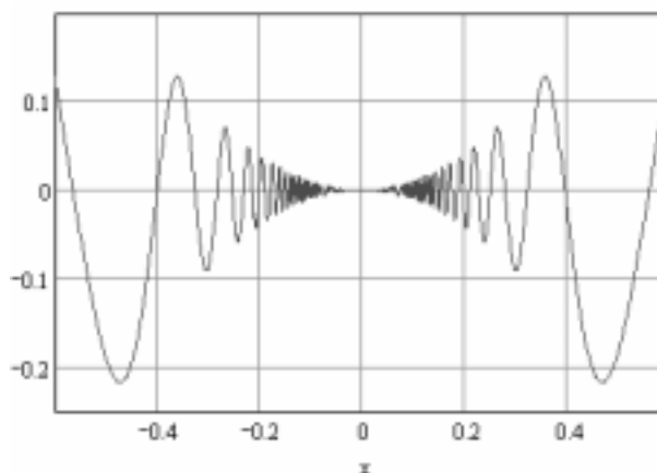
Рис. 1. График функции
